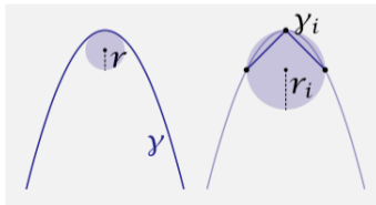
Соприкасающаяся окружность
